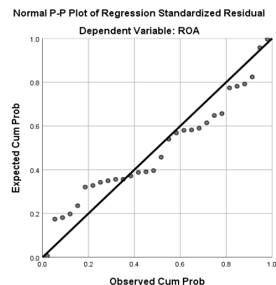
Gambar 1. Uji normalitas
