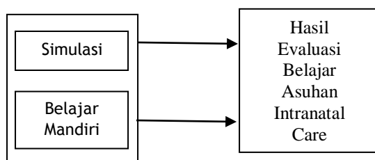
Gambar 1. Kerangka Konsep
